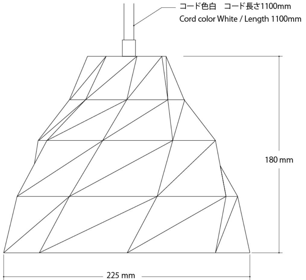
正面図 / Front view
